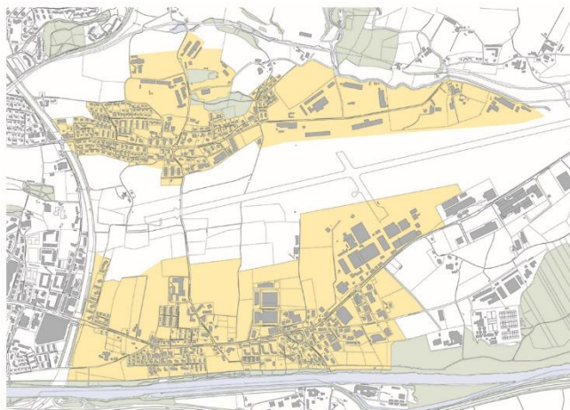
Geplanter Ausbau der Fernwärmeversorgung für Emmen Dorf und Armasuisse
